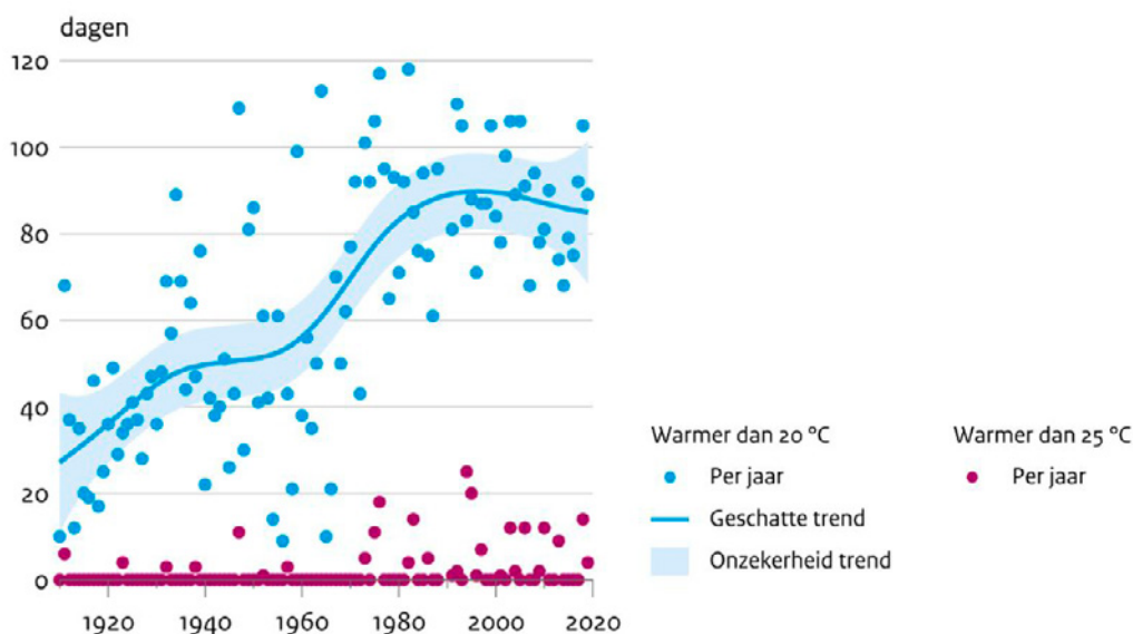
Figuur 2-2: Maaswater Eijsden en Borgharen: aantal dagen met een temperatuur hoger dan 20°C en 25°C (bron: Compendium voor de Leefomgeving 2020).
